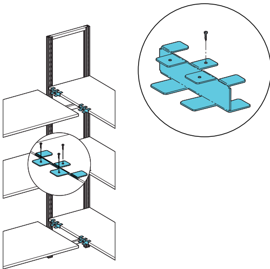
KRIŽNO UČVRŠČENJE
