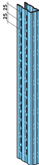
PROFIL STANDARDNOG STUPA
