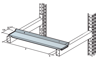
DRŽAČ KONTEJNERA
