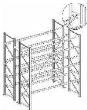
KRIŽNA UČVRŠĆENJA
