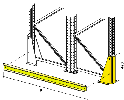
VERTIKALNI I HORIZONTALNI ŠTITNIK STUPA BOČNE STRANE
